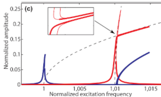
Diagramme de stabilité pour un nanofil avec couplage non linéaire entre polarisations
